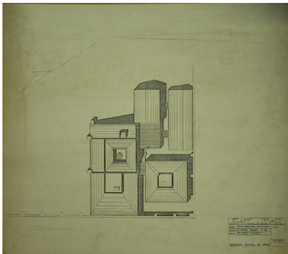
Figura 58. Plano de planta de techos, propuestas de mejoramiento del Centro Universitario Los Belenes. DGA UAEM.
