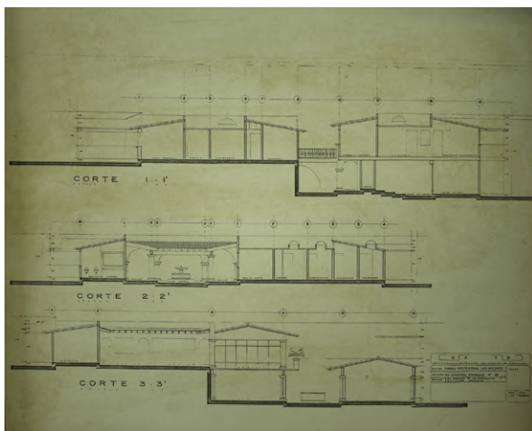
Figura 57. Plano de cortes longitudinales por fachada de las propuestas de remodelación del Centro Universitario Los Belenes en la década de los ochenta. DGA UAEM.
