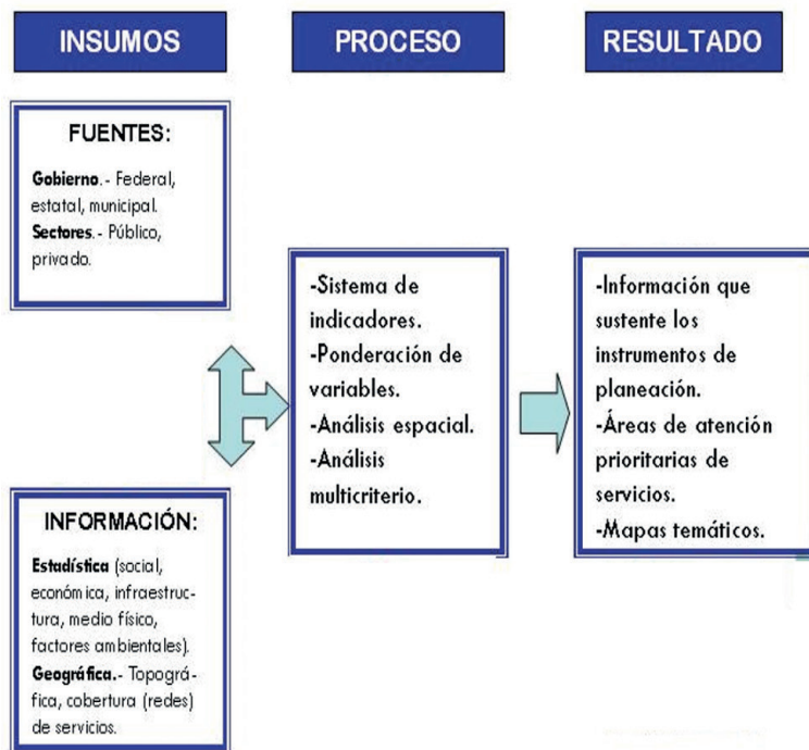
Figura 2. Síntesis gráfica de la metodología utilizando un SIG. 2010.
